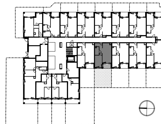
SCHEMAT KONDYGNACJI
